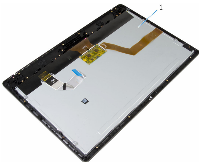
1 顯示器組件
